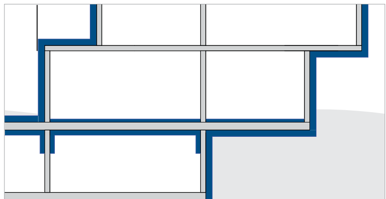
Gebräuchliche Dämmung mit Unterdecken- und Flankendämmung
