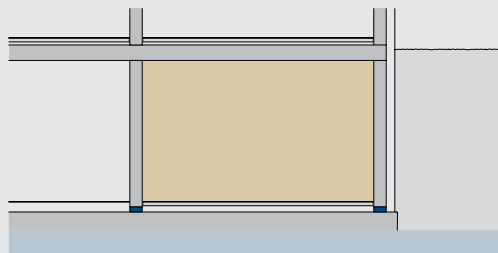
Bodenplattenlösung Waschraum / Sauna
