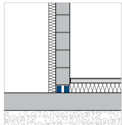
Sconnex® Typ M
