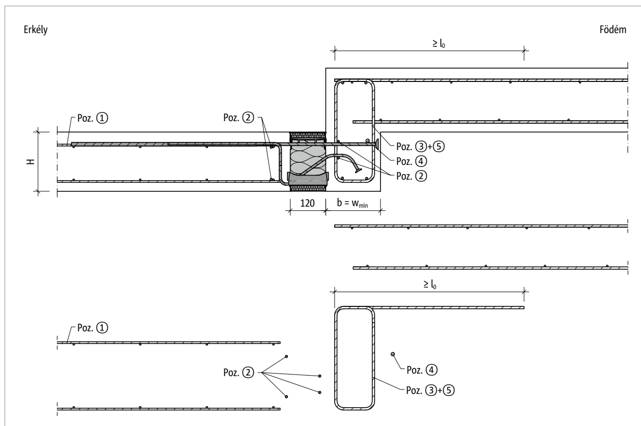
Ábra 94: Schöck Isokorb® XT KL-U típus: Helyszíni vasalás - erkély lefelé födémugrással, minimális szerkezeti elemmérettel ( w_{\text{tényl}} = w_{\min} )
