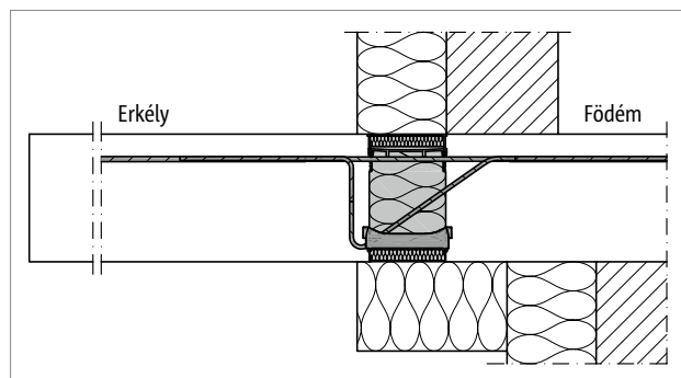
Ábra 25: Schöck Isokorb® XT KL típus: Csatlakozás közvetett alátámasztási födém és hőszigetelő rendszer esetén
