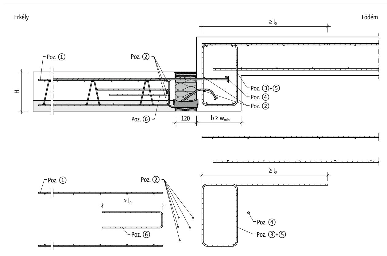
Ábra 108: Schöck Isokorb® XT KL-U-F típus: Helyszíni vasalás, lefelé földemugrásos erkély
