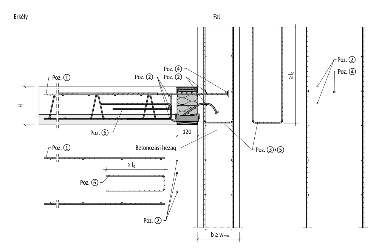
Ábra 109: Schöck Isokorb® XT KL-U-F típus: Helyszíni vasalás, felfelé földemugrásos erkély
