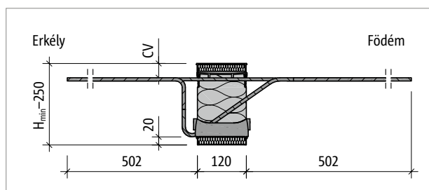
Ábra 35: Schöck Isokorb® XT KL-M5, M6 típus: termékmetszet
