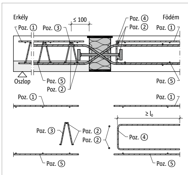
Ábra 167: Schöck Isokorb® XT QP-VV típus: Helyszíni vasalás, erkélyoldalon rácsos borda esetén
