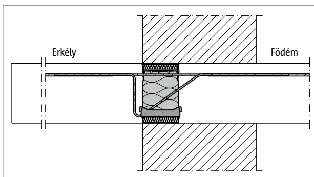
Ábra 24: Schöck Isokorb® XT KL típus: Csatlakozás egyhéjú falazatnál
