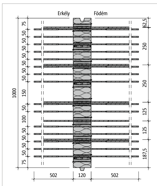
Ábra 37: Schöck Isokorb® XT KL-M6 típus: termék alaprajz
