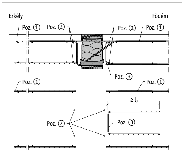
Ábra 47: Schöck Isokorb® XT KL típus: Helyszíni vasalás közetett alátámasztásnál
