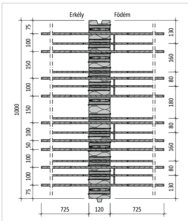
Ábra 40: Schöck Isokorb® XT KL-M8 típus: termék alaprajz
