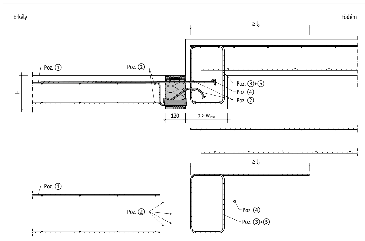
Ábra 95: Schöck Isokorb® XT KL-U típus: Helyszíni vasalás - erkély lefelé födémugrással, nagyobb építőelem mérettel ( w_{\text{tényl}} > w_{\min} )
