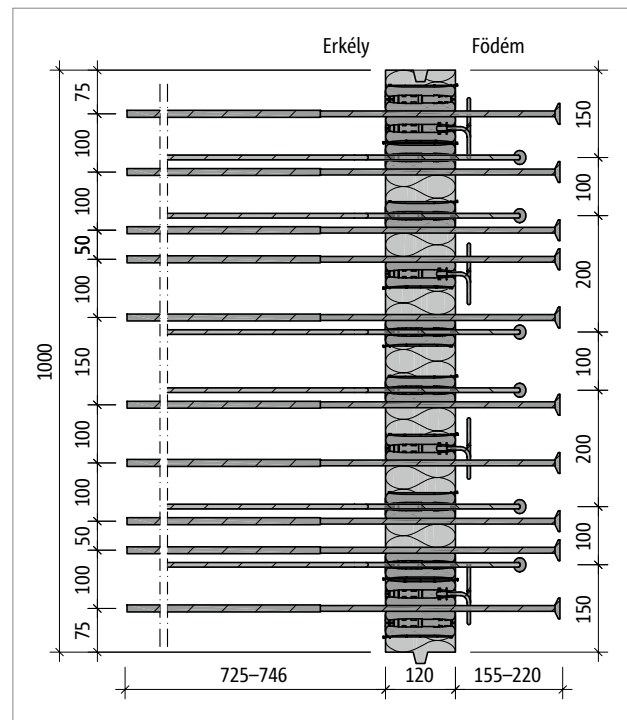
Ábra 88: Schöck Isokorb® XT KL-U-M4 típus: termék alaprajz
