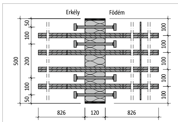
Ábra 163: Schöck Isokorb® XT QP-VV9 típus: termék alaprajz
