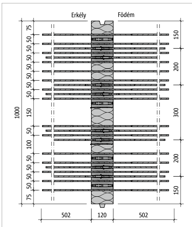
Ábra 41: Schöck Isokorb® XT KL-M5-VV1 típus: termékalaprajz
