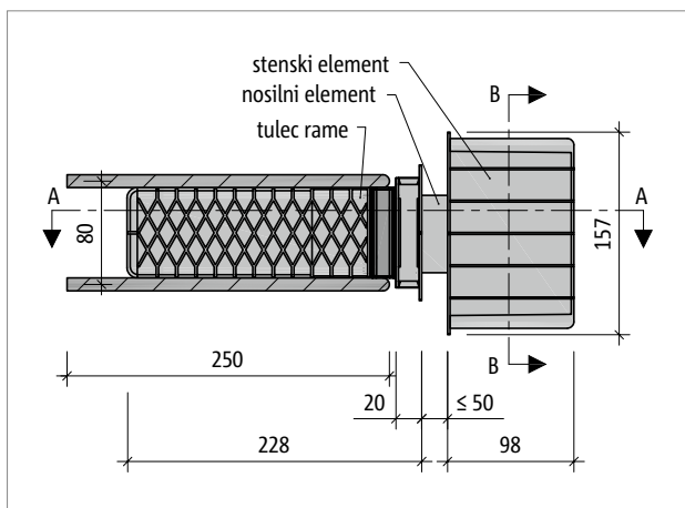
Sl. 84: Schöck Tronsole® tip Q: tloris proizvoda
