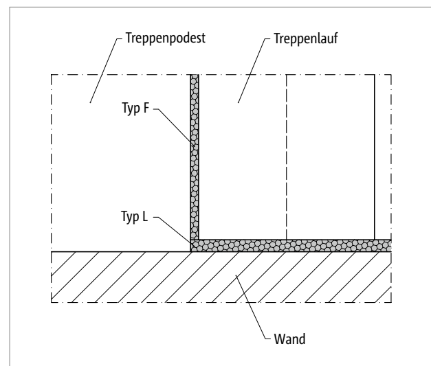
Abb. 65: Schöck Tronsole® Typ F: Elementanordnung, Detail B
