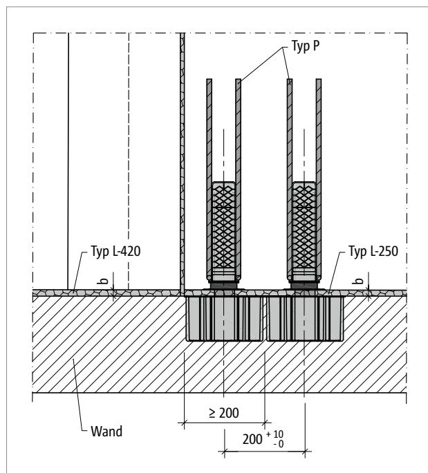
Abb. 125: Schöck Tronsole® Typ P (paarweise Anordnung): Elementanordnung, Detail C, Fugenbreite b = 15 \text{ mm} bei Ortbeton, bei Fertigteiltreppenhäufen ist die Notwendigkeit einer zusätzlichen Einbautoleranz durch den Planer zu prüfen
