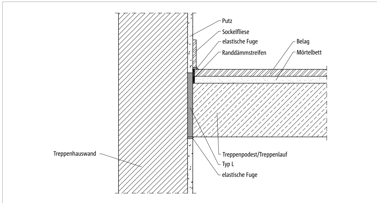
Abb. 187: Schöck Tronsole® Typ L: Einbauschnitt Ortbetontreppe
