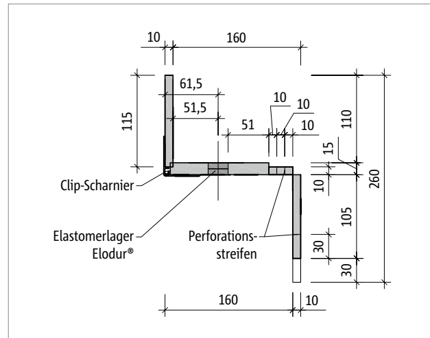
Abb. 71: Schöck Tronsole® Typ F-V1, F-V2, F-V3: Produktschnitt, Schnitt A-A bei Anpassung an die maximale Konsoltiefe
