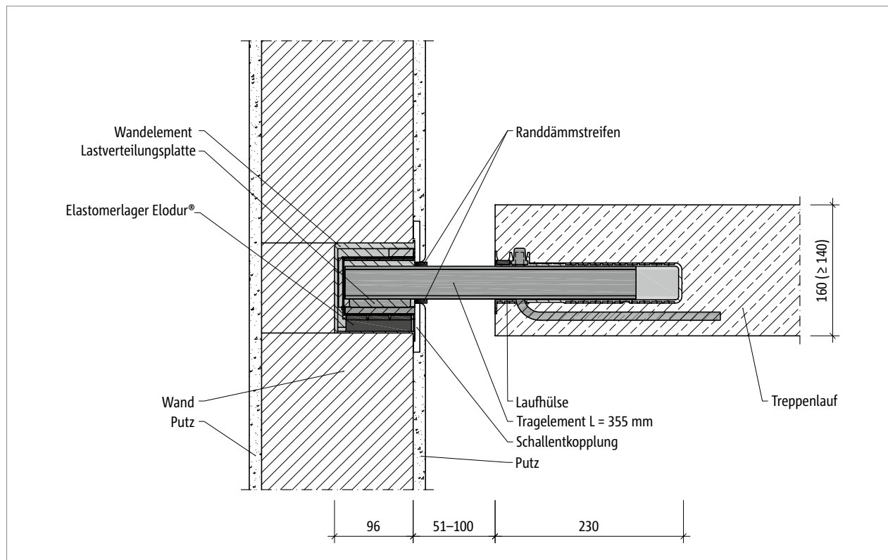
Abb. 91: Schöck Tronsole® Typ Q-FV-XL oder Q-A2-XL: Einbauschnitt
