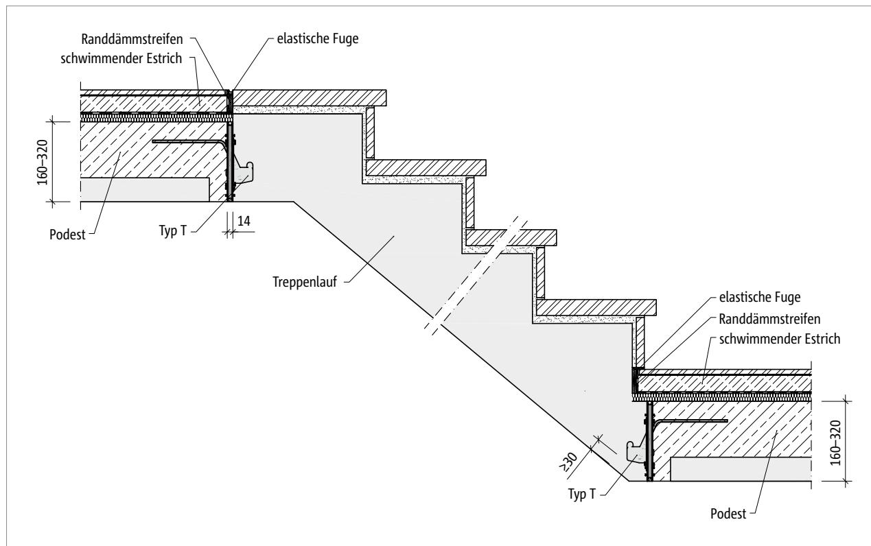
Abb. 25: Schöck Tronsole® Typ T: Einbauschnitt Fertigteilstufe mit Halbfertigteilpodest
