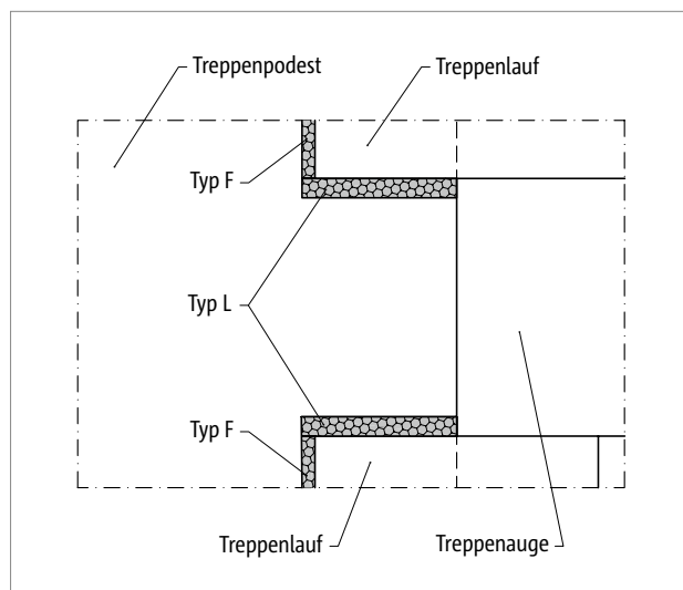
Abb. 64: Schöck Tronsole® Typ F: Elementanordnung, Detail A
