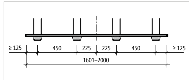
Abb. 39: Schöck Tronsole® Typ T-V4-...-L1601 bis L2000: Produktgrundriss
