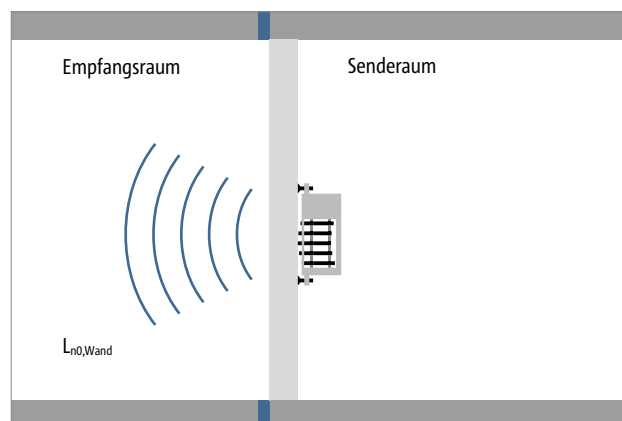
Abb. 8: Bestimmung des Norm-Wand-Trittschallpegels L_{n0,Wand} der Referenzwand im Prüfstand
