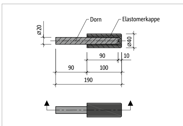
Abb. 178: Schöck Tronsole® Typ D: Produktgrundriss
