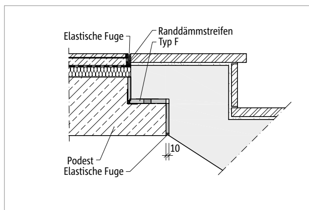
Abb. 15: Schöck Tronsole® Typ F: Brandschutzausführung
