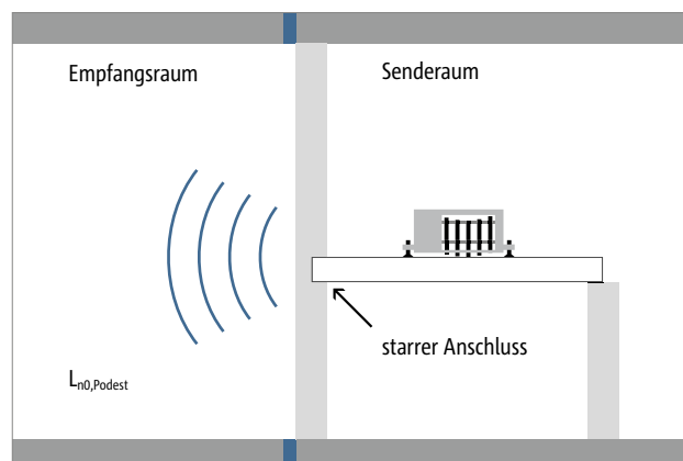
Abb. 10: Bestimmung des Norm-Podest-Trittschallpegels L_{n0,Podest} des Referenzpodests ohne Trittschalldämmelement
