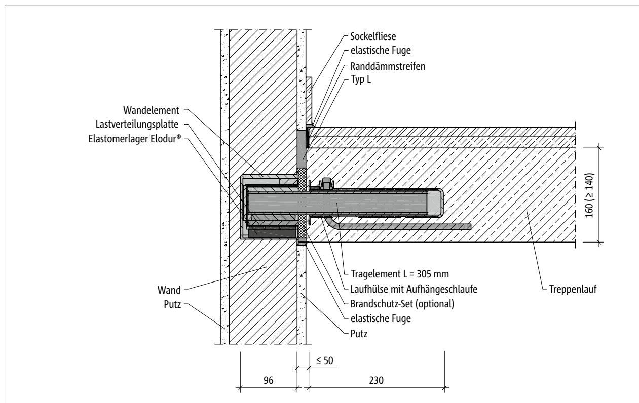
Abb. 90: Schöck Tronsole® Typ Q-FV oder Q-A2: Einbauschnitt Wanddicke 11,5 cm
