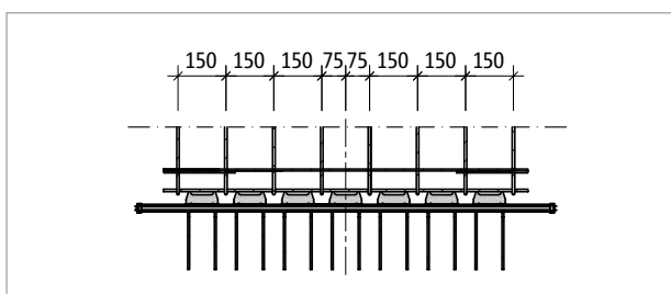
Abb. 50: Schöck Tronsole® Typ T: Vershobenes Verlegeraster der Bewehrung bei ungerader Anzahl von Tragkonsolen an der Tronsole®
