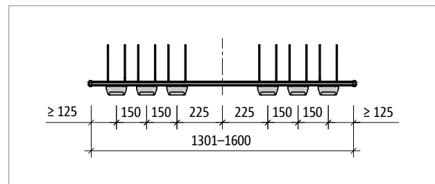
Abb. 41: Schöck Tronsole® Typ T-V6-...-L1301 bis L1600: Produktgrundriss
