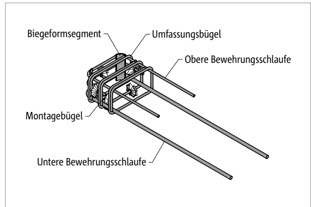
Schöck Tronsole® Typ Z Part T
