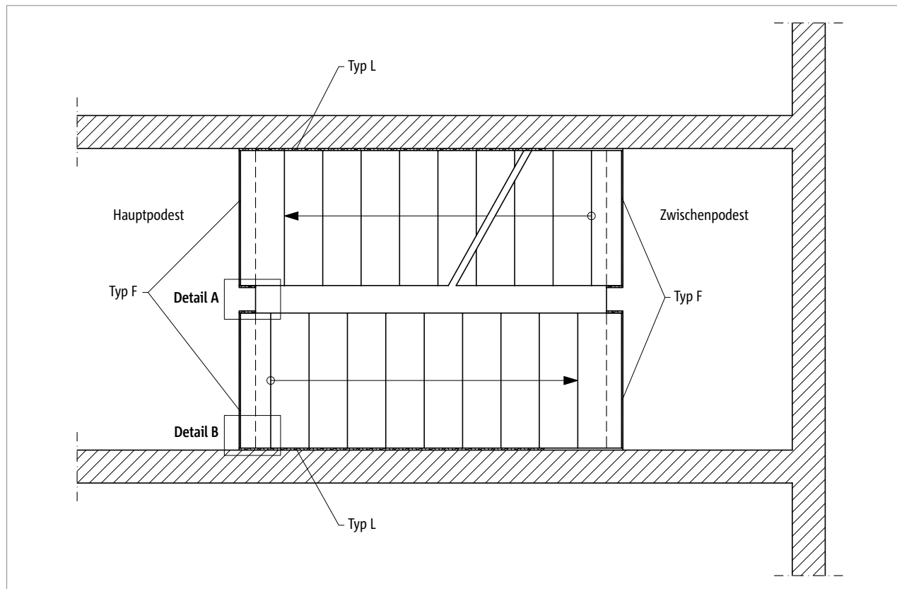
Abb. 63: Schöck Tronsole® Typ F: Elementanordnung im Grundriss
