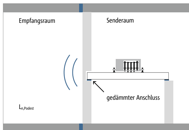
Abb. 9: Bestimmung des Norm-Podest-Trittschallpegels L_{n,Podest} des Referenzpodests mit zu prüfendem Trittschalldämmelement
