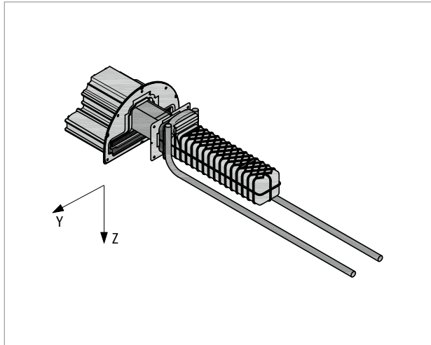
Abb. 130: Schöck Tronsole® Typ P: 3D-Ansicht mit Achsbezeichnung
