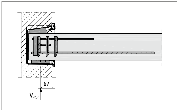
Abb. 163: Schöck Tronsole® Typ Z: Darstellung der Wirkungslinie der Auflagerkraft in der Wand
