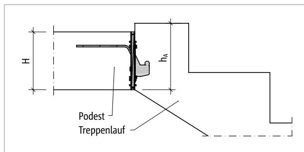
Abb. 47: Schöck Tronsole® Typ T: Anschlusshöhe h_A
