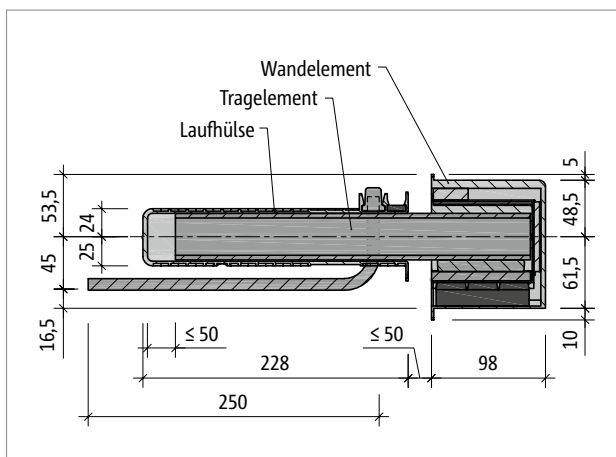
Abb. 100: Schöck Tronsole® Typ Q: Produktschnitt A-A
