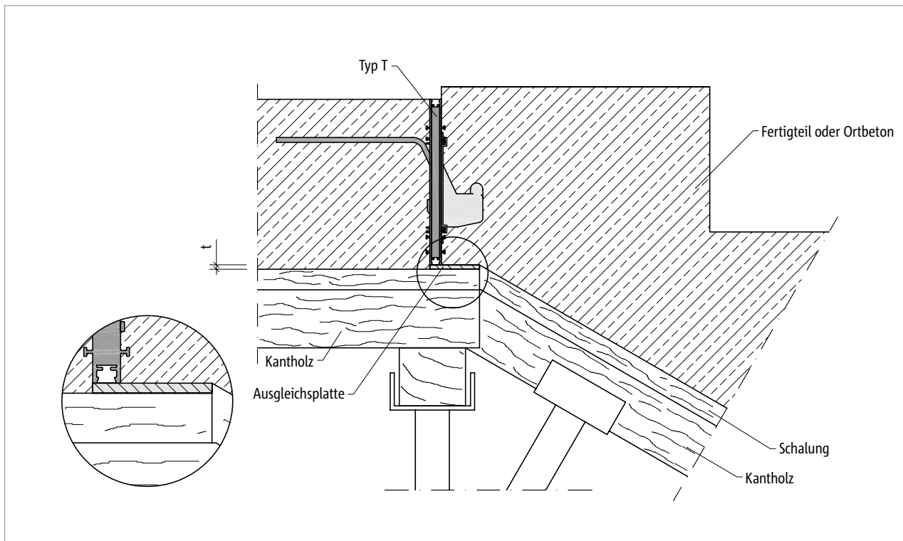
Abb. 55: Schöck Tronsole® Typ T: Berücksichtigung der Einfederung des Treppenlaufs mittels bauseitiger Ausgleichsplatte der Dicke t
