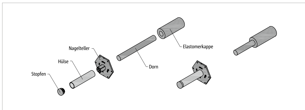
Abb. 168: Schöck Tronsole® Typ D-H
