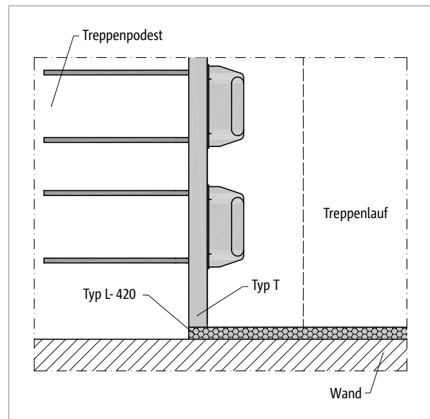
Abb. 28: Schöck Tronsole® Typ T: Elementanordnung Detail B
