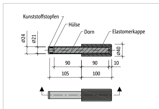
Abb. 179: Schöck Tronsole® Typ D-H: Produktgrundriss
