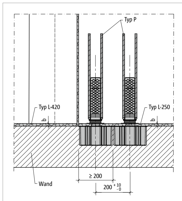
Abb. 125: Schöck Tronsole® Typ P (paarweise Anordnung): Elementanordnung, Detail C, Fugenbreite b = 15 \text{ mm} bei Ortbeton, bei Fertigteiltreppeläufen ist die Notwendigkeit einer zusätzlichen Einbautoleranz durch den Planer zu prüfen
