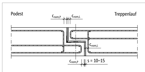
Abb. 166: Schöck Tronsole® Typ F: Vertikalschnitt längs der Treppe im Bereich des Konsolaufagers; Darstellung der Betondeckung c_{nom,L} und c_{nom,P}
