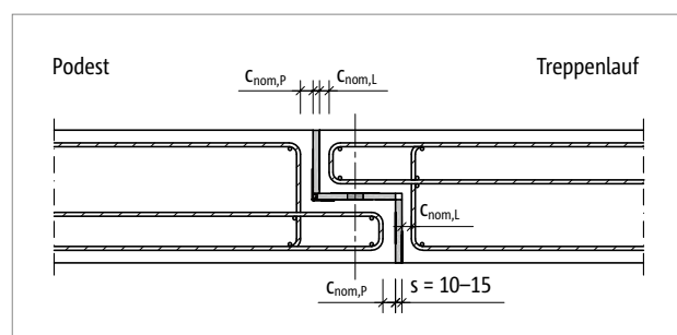
Abb. 157: Schöck Tronsole® Typ F: Vertikalschnitt längs der Treppe im Bereich des Konsolauflagers; Darstellung der Betondeckung c_{nom,L} und c_{nom,P}
