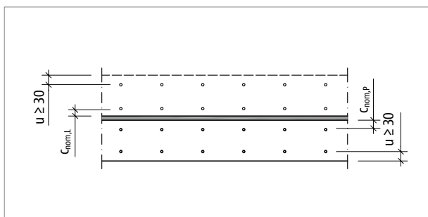
Abb. 167: Schöck Tronsole® Typ F: Vertikalschnitt quer zur Treppe im Bereich des Konsolaufagers; Darstellung der Betondeckung c_{nom,L} , c_{nom,P} und des Mindestachsabstandes u der Bewehrung
