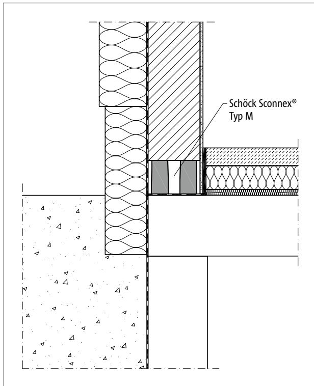
Abb. 251: Schöck Sconnex® Typ M: Einbauzustand bei Wärmedämmverbundsystem
