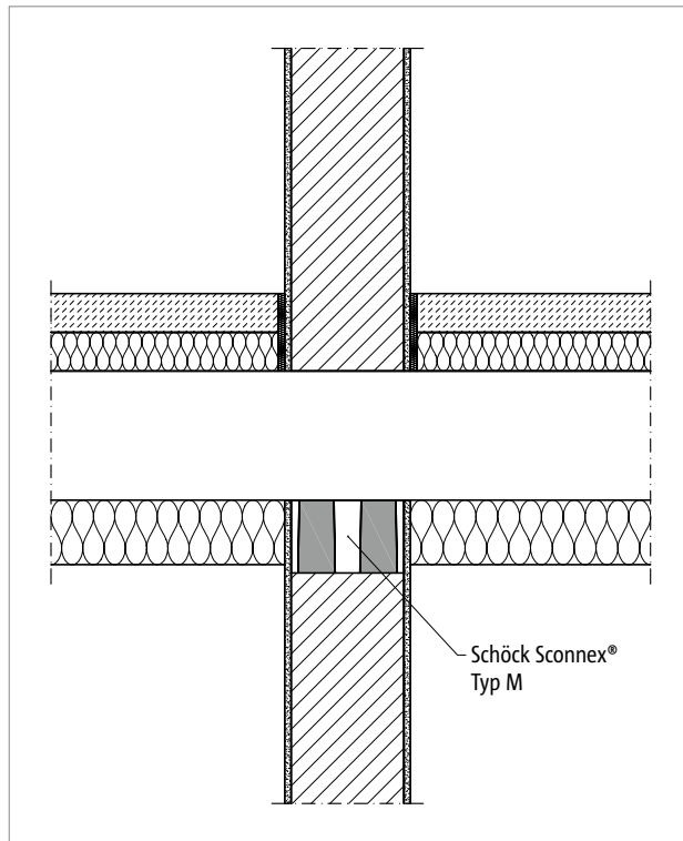
Abb. 255: Schöck Sconnex® Typ M: Einbauzustand bei Innenwand und Unterdeckendämmung
