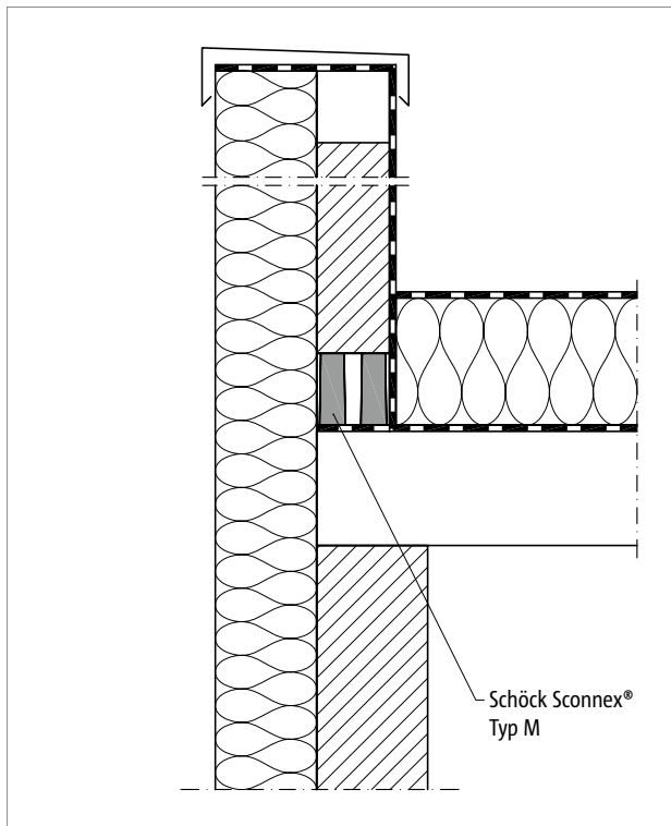
Abb. 253: Schöck Sconnex® Typ M: Einbauzustand in der Attika
