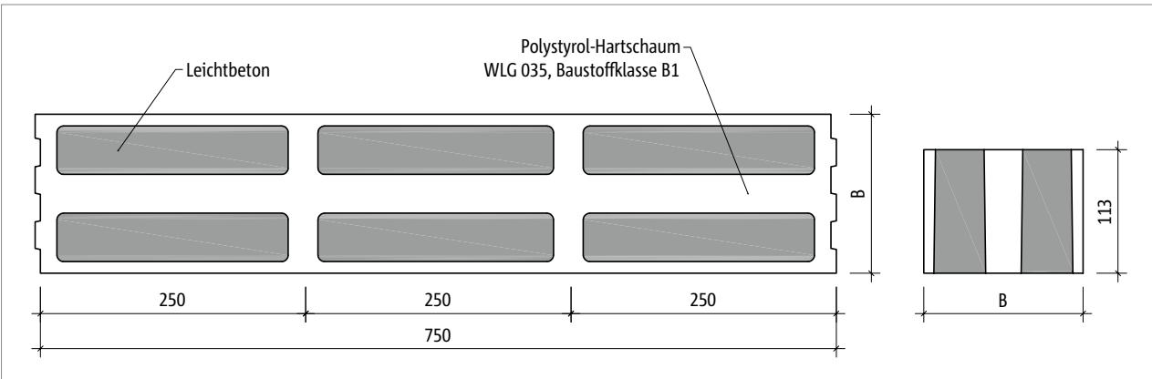
Abb. 257: Schöck Sconnex® Typ M: Abmessungen
