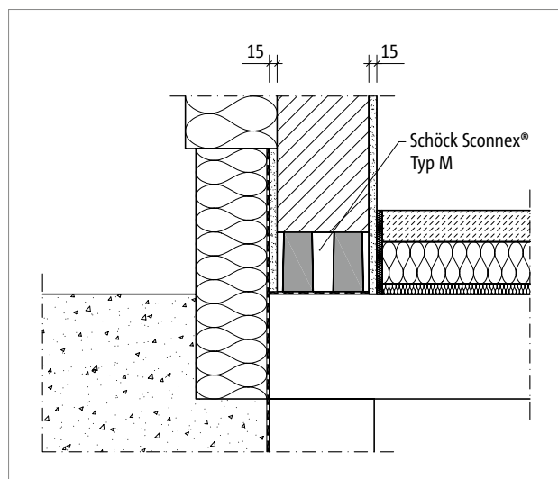
Abb. 258: Schöck Sconnex® Typ M: REI 30 bzw. REI 90 Ausbildung bei brandschutztechnischem Raumabschluss
