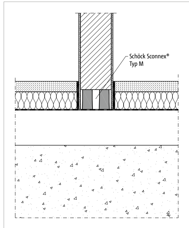
Abb. 256: Schöck Sconnex® Typ M: Einbauzustand bei Innenwand auf Bodenplatte
